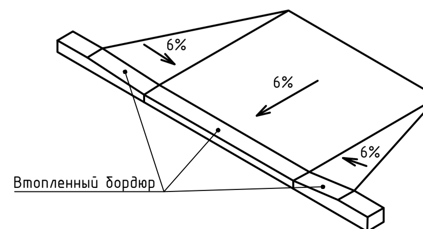
Схема устройства пандуса из тротуарной плитки
